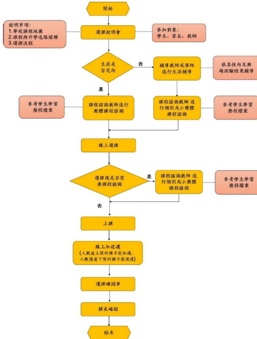
※選課流程圖
